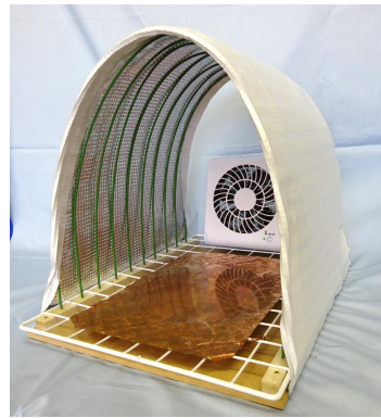
広島県産業教育振興会会長賞 「なんでも常温機」 広島大学附属福山中学校 第1学年の作品
