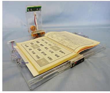
広島県知事賞 「寝落ち対応自動しおり・ 消灯機能付き読書灯」 広島大学附属福山中学校 第2学年の作品
